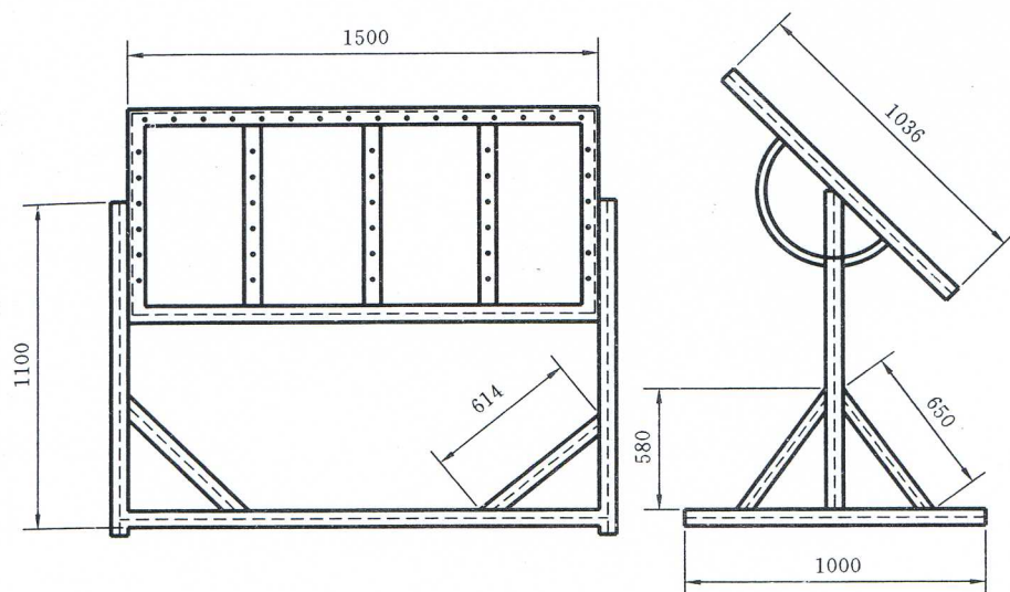
图2 可调角度的曝露架
